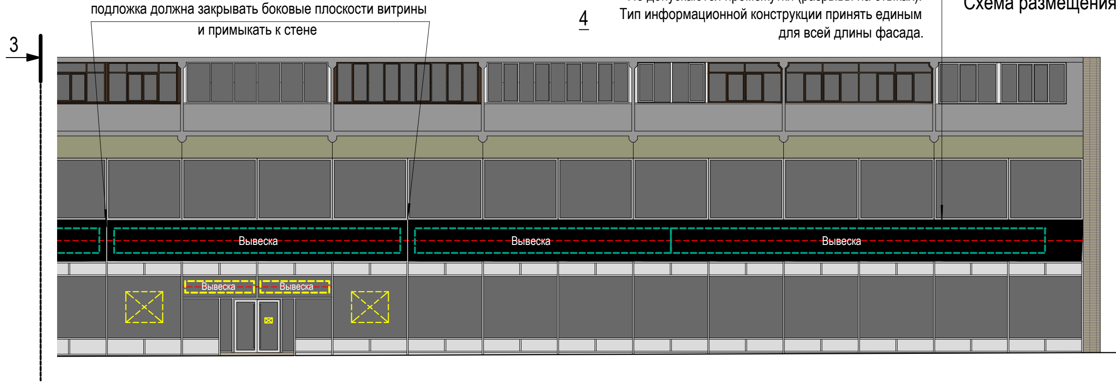
Схема размещения
