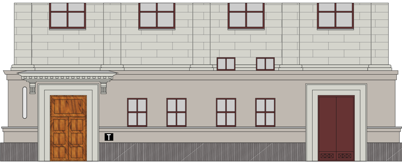
Схема размещения
