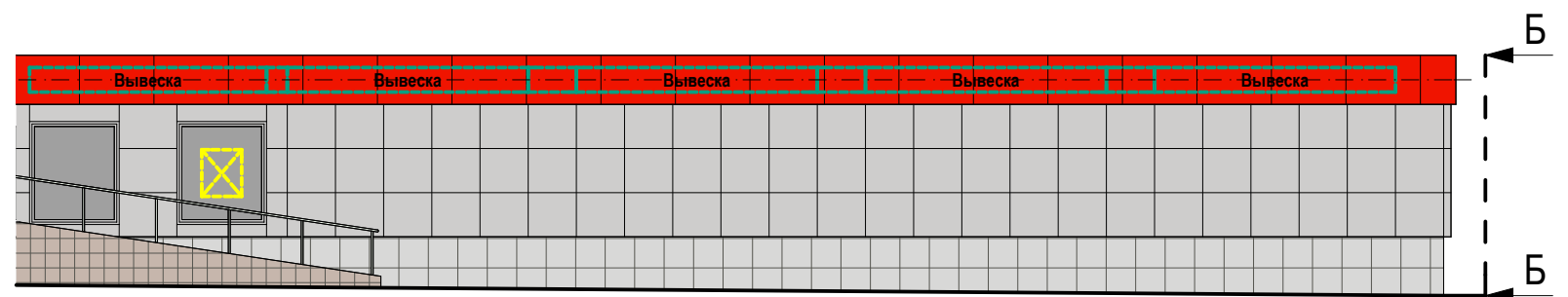
Схема размещения
