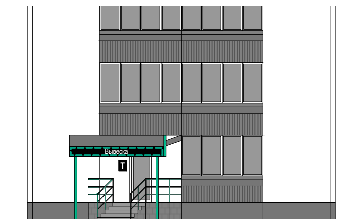
2 Схема размещения
